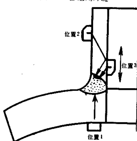
图 19 管座角焊缝
