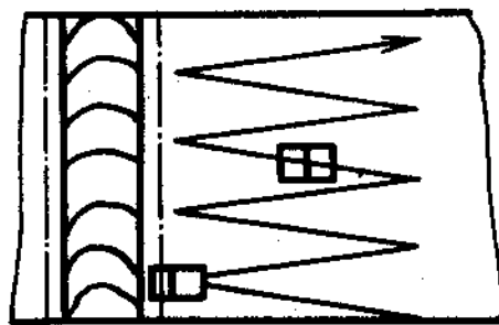
图 11 锯齿形扫查
